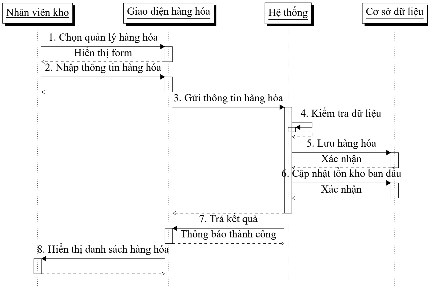
Hình 1: Sequence diagram UC05 – Quản lý hàng hóa
